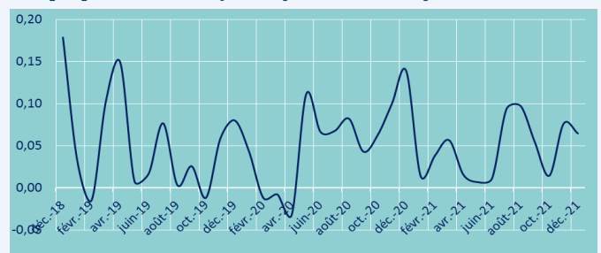
Graphique : Indicateur synthétique des soldes d'opinion
